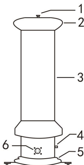
图 3 倍压筒示意图
