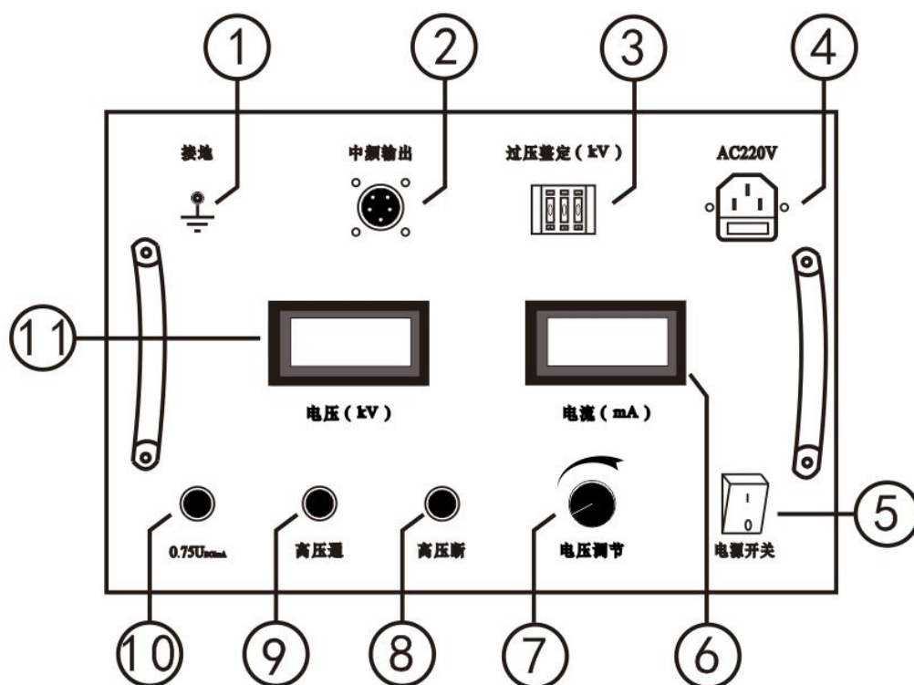
图2 面板布局图
