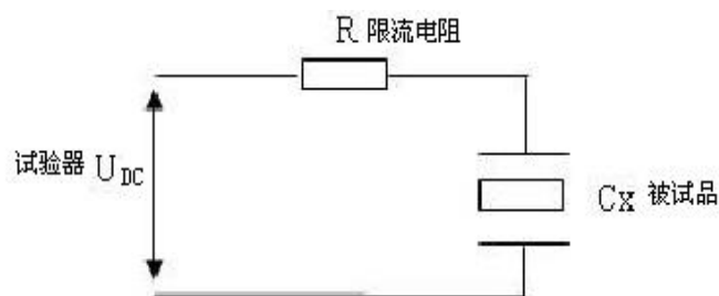
图 9 限流电阻使用示意图
